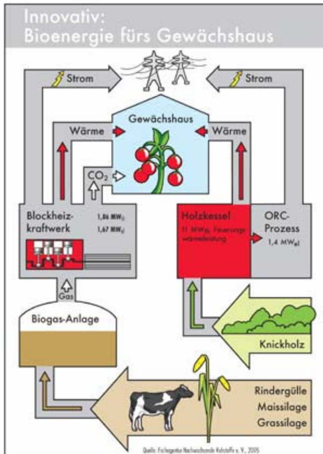
Abbildung 76: Wärmenutzung aus Biogasanlage/Holzkessel durch Gewächshausbetrieb in Hennstedt 299
