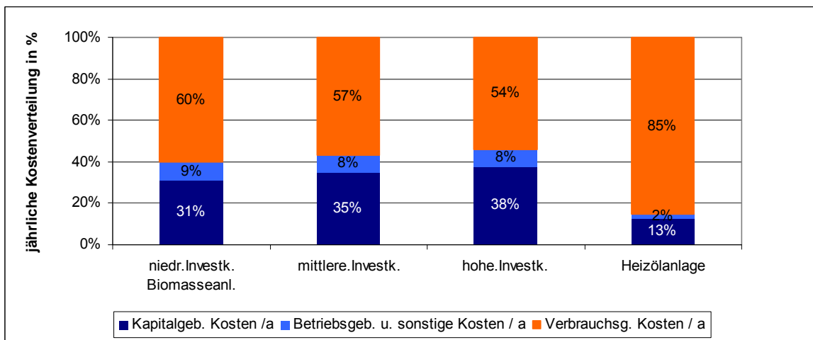
Abbildung 89: Kostenverteilung der jährlichen Gesamtkosten einer Holzhackschnittelheizung bei unterschiedlicher Investitionskostenhöhe im Vergleich zu einer Heizölanlage/Kalthaus 2 500 m 2
