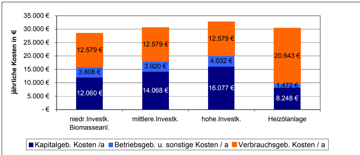
Abbildung 91: Kostenverteilung der jährlichen Gesamtkosten einer Kohleheizanlage bei unterschiedlicher Investitionskostenhöhe im Vergleich zu einer Heizölanlage/Kalthaus 2 500 m 2
