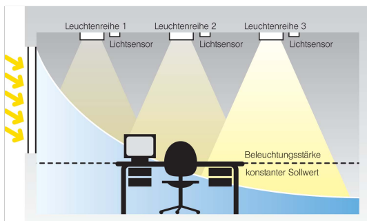
Bild 4: Konstantlichtregelung mit dimmbaren EVG (Quelle: Fördergemeinschaft Gutes Licht)
