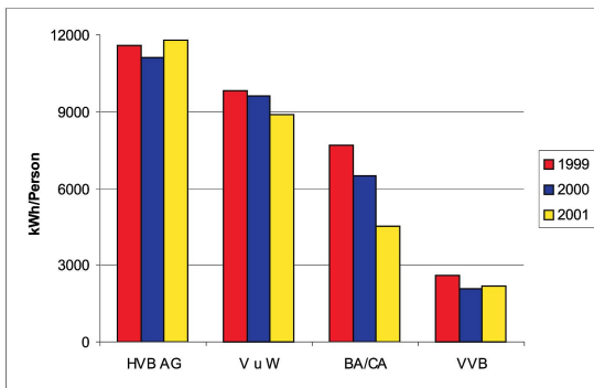
Bild 2: Spezifischer Stromverbrauch von Bürogebäuden der HVB Group. (Quelle: Nachhaltigkeitsbericht HVB Group 2002)
