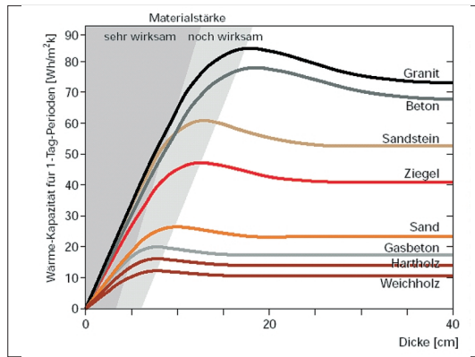
Bild 8: Speicherwirkung von Bauteilen: Einfluss des Materials und der Einbaustärken (Quelle: Wuppertal Institut)
