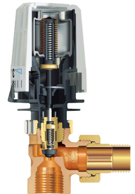
Bild 12: Längsschnitt durch ein Thermostatventil (Quelle: Fa. Heimeier)
