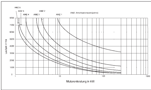
Bild 7: Einfache Abschätzung der Wirtschaftlichkeit durch Ventilatortausch (Quelle: Landesgewerbeamt Ba-Wü)
